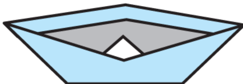
10. TA DAAA!
